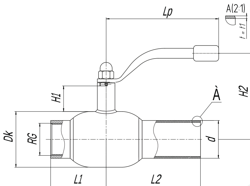
КШГ Серия 12, DN 15–50, PN 4,0 МПа Резьба / Сварка
