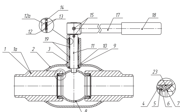
DN 65–100
