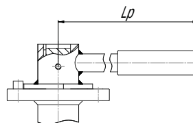
КШГ Серия 15, DN 100–400, PN 1,6/2,5 МПа Фланец/Фланец
