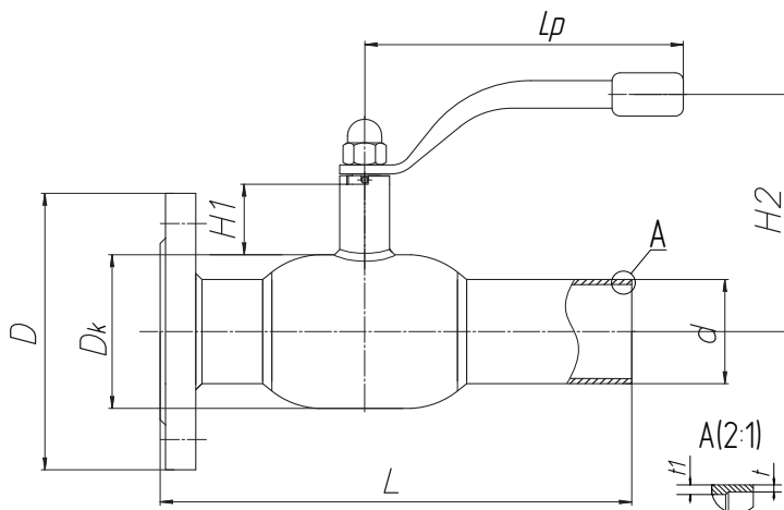
КШГ Серия 12, DN 20–150, PN 2,5/4,0 МПа Фланец/Сварка
