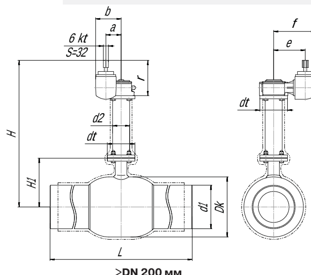
КШГ Серия 32, DN 32–600*, PN 2,5/4,0 МПа
