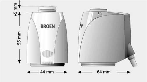
Рис. 49 Габаритные размеры привода
