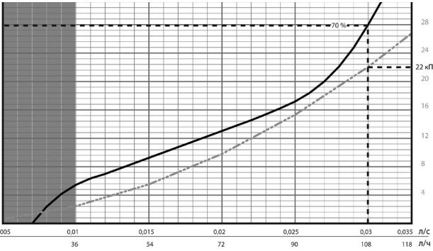
Рис. 40 Диаграмма для клапана БРОЕН Dynamic DN15 Low (артикул 4360000L-000001)
