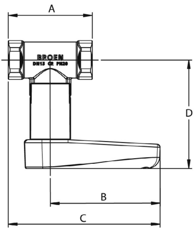
Рис. 17 Клапан БРОЕН Venturi DRV DN15-050 муфтовый
