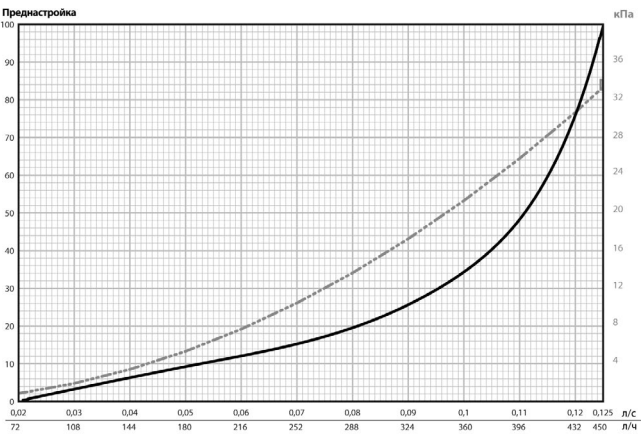
Рис. 41 Диаграмма для клапана БРОЕН Dynamic DN15 Standart (артикул 4360000S-000001)
