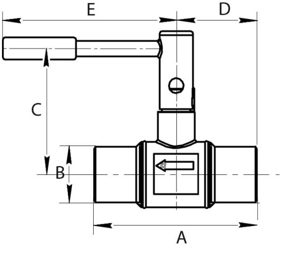
Рис. 23 Клапан БРОЕН Venturi DRV DN 065-200 под приварку
