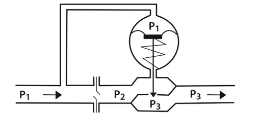
Рис. 32 Физическая модель работы функции автоматического ограничения расхода на клапане БРОЕН Dynamic
