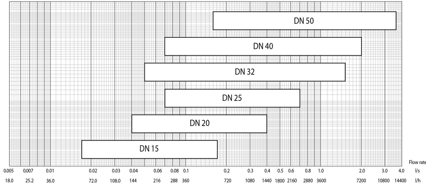
Номограмма для определения типоразмера клапана БРОЕН V
