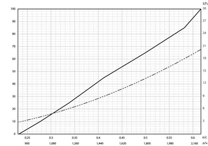
Рис. 44 Диаграмма для клапана БРОЕН Dynamic DN20 High (артикул 4460000H-000001)
