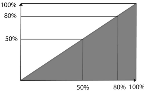
Рис. 34 Теоретическая зависимость расхода от степени открытия клапана БРОЕН Dynamic
