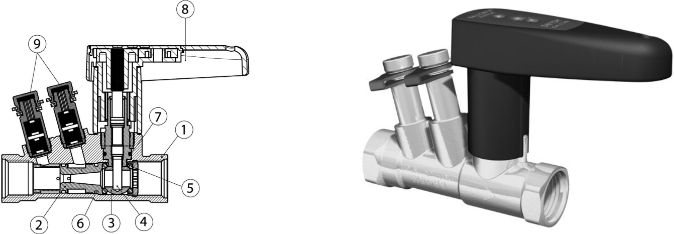
Рис.3 Спецификация материалов статического балансировочного клапана БРОЕН Venturi DN10-50
