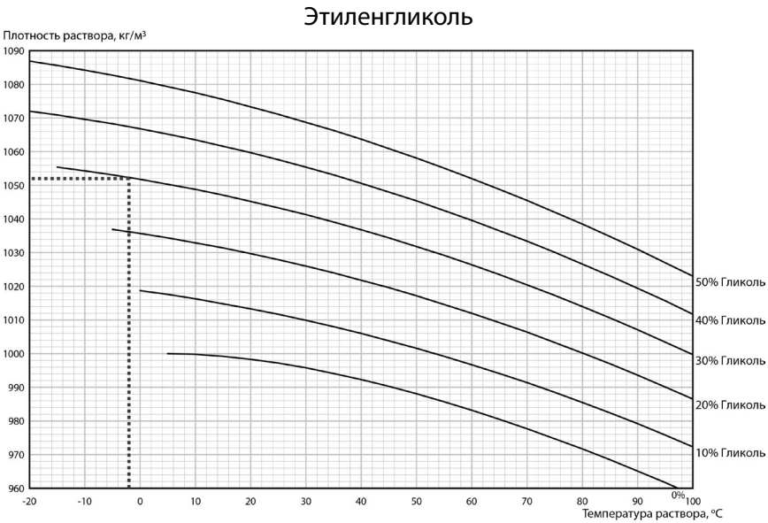
Рис. 64 График зависимости плотности водного раствора этиленгликоля от температуры и концентрации
