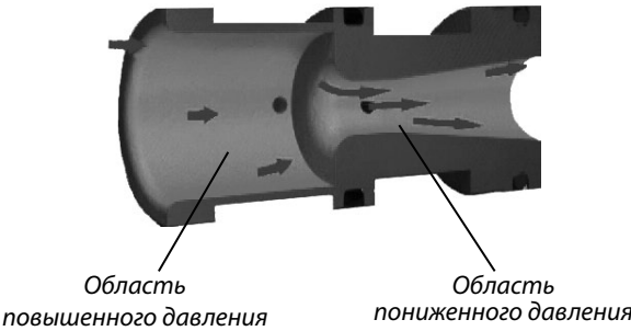
Рис. 36 Конструкция измерительной диафрагмы клапана БРОЕН Dynamic
