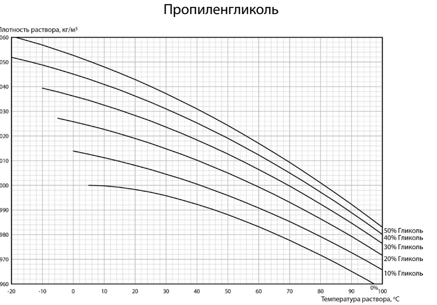
Рис. 65 График зависимости плотности водного раствора пропиленгликоля от температуры и концентрации
