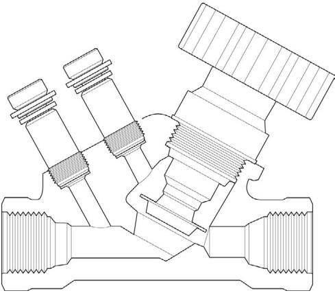
Рис. 5 Седельчатая конструкция клапана
