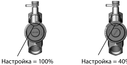
Рис. 39 Грубая настройка клапана БРОЕН Dynamic на расчетный расход (без расходомера)
