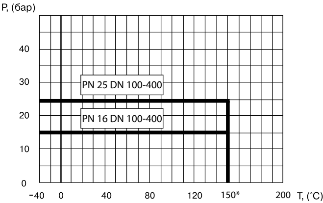
Зависимость «Температура-Давление»
