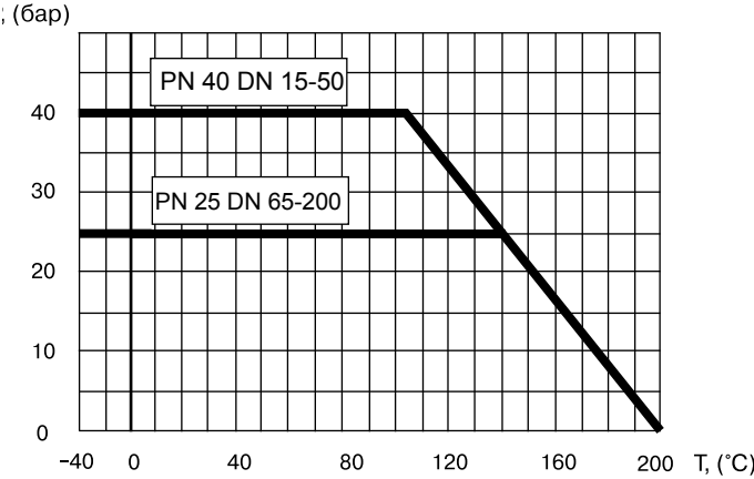
Зависимость «Температура-Давление»
