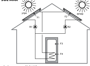
Схема №5 SOL MAX
