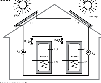
Схема №6 SOL MAX
