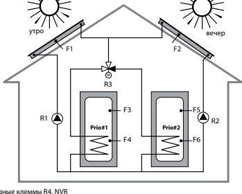
Схема №7 SOL MAX
