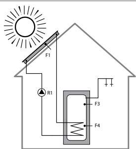
Схема №1 SOL MAX SOL BASIS
