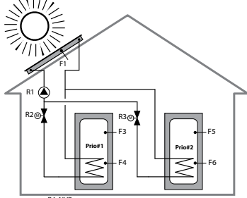
Схема №7 SOL MAX
