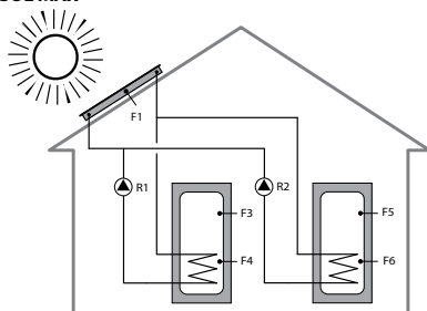
Схема №2 SOL MAX
