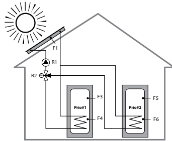
Схема №3 SOL MAX
