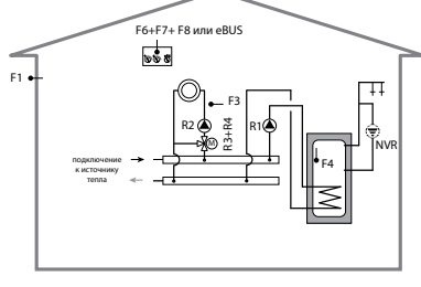
Схема №7 HZR-C HZR-E*
