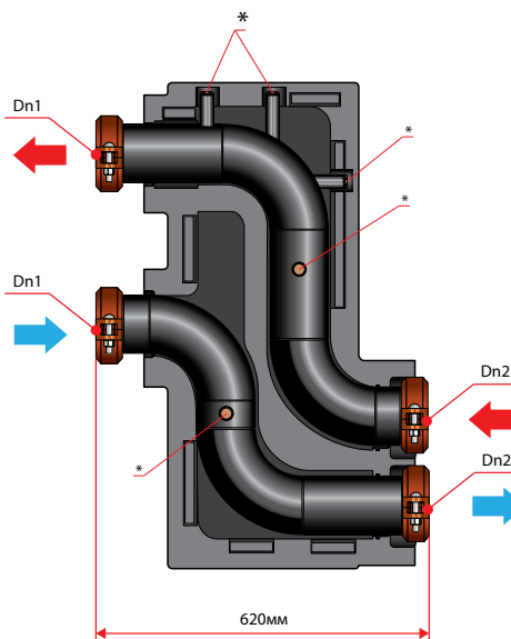
Подключение гидрострелка/каскадный коллектор
