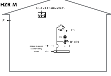
Схема №8 HZR-C HZR-E* HZR-M
