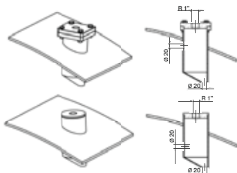
Пример патрубка. Внутренняя установка в котел
