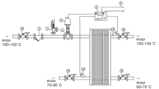
Погодозависимая схема регулирования
