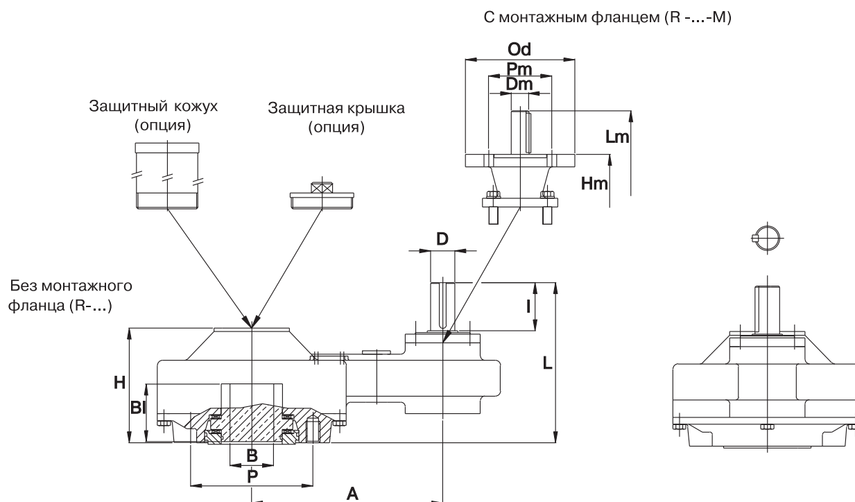
Габаритные и присоединительные размеры редукторов с монтажным ISO-фланцем
