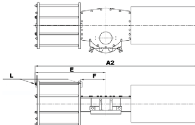
С возвратной пружиной PD-S
