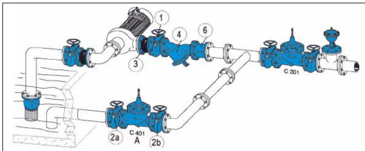
Рис. 1 Пример установки регулятора давления C101.
