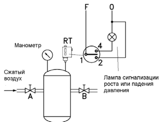
Рис. 9. пример использование реле давления с нейтральной зоной
