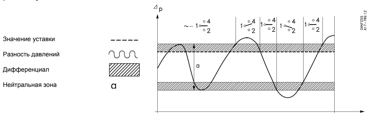
Рис. 12. Принцип действия реле давления с выключателями SPDTNP.
