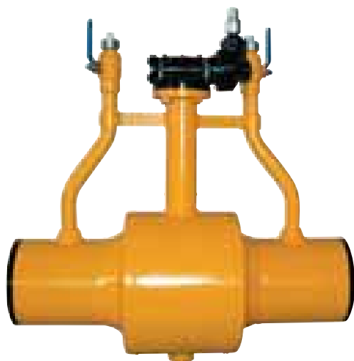
Штампованные шаровые краны с двумя дренажами
