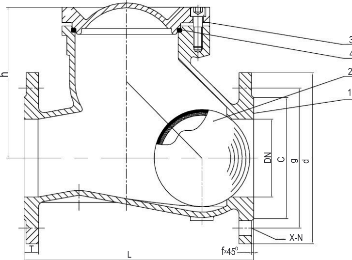
Чертеж габаритный обратного клапана для канализации шарового фланцевого ABRA-D-022-NBR (размеры в таблице ниже):
