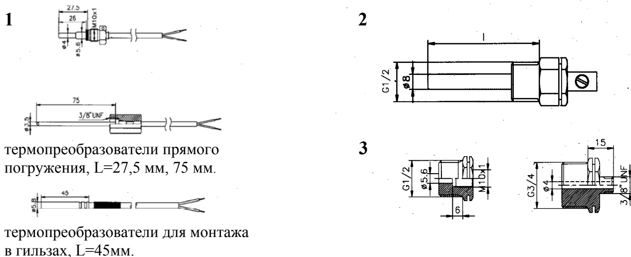
Рисунок 2. Термопреобразователи сопротивления.
