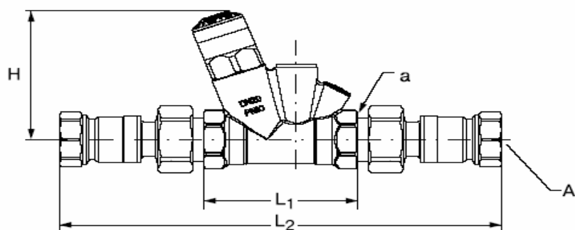
Рис. 4. Габаритные и присоединительные размеры клапана MTCV. (Взято из RC.08.A6.50)
