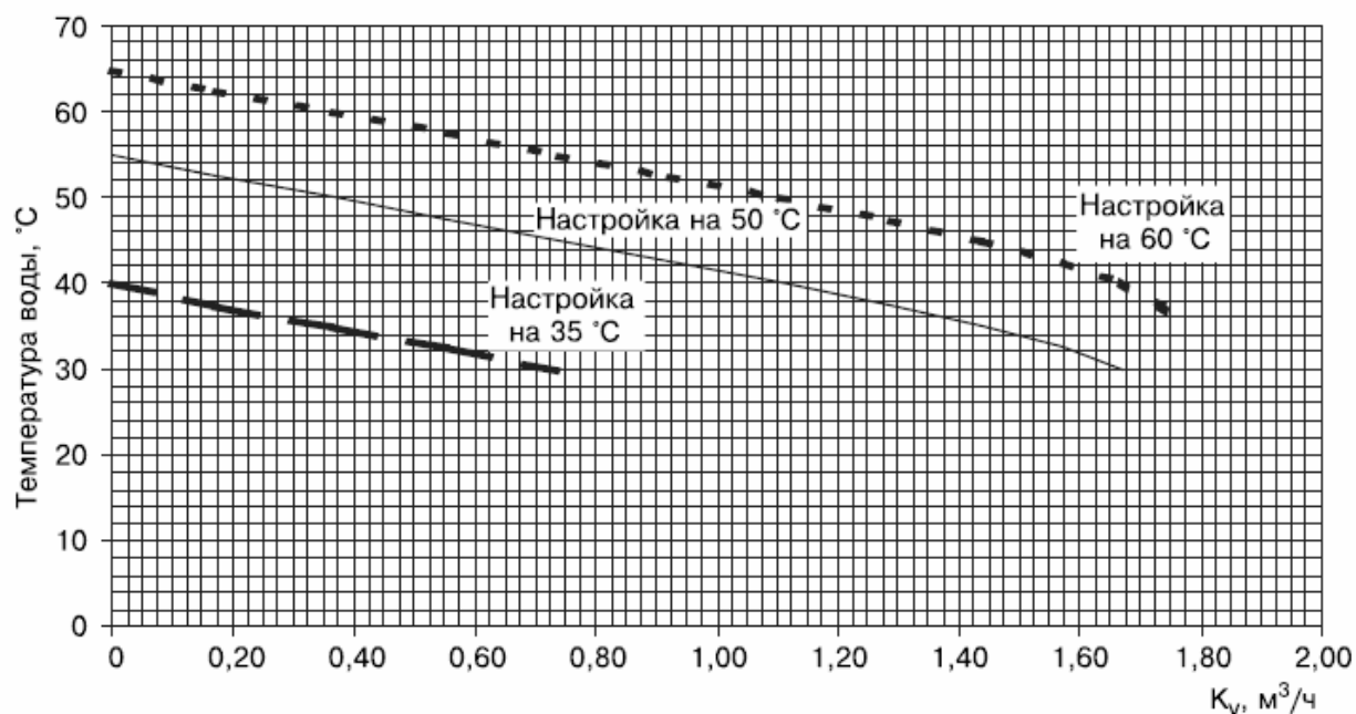
Рис. 7. Зависимость K_v клапана MTCV, D_y=20 мм, от его настройки и температуры воды. (Взято из RC.08.A6.50)
