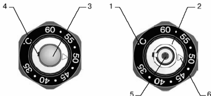
Рис. 7. Температурная настройка клапана MTCV: 1 – шкала температурной настройки; 2 – кольцо настройки; 3 – заглушка настроечного винта; 4 – отверстие для удаления заглушки; 5 – отверстие в винте настройки под шестигранный ключ; 6 – метка температурной настройки. (Взято из RC.08.A6.50)
