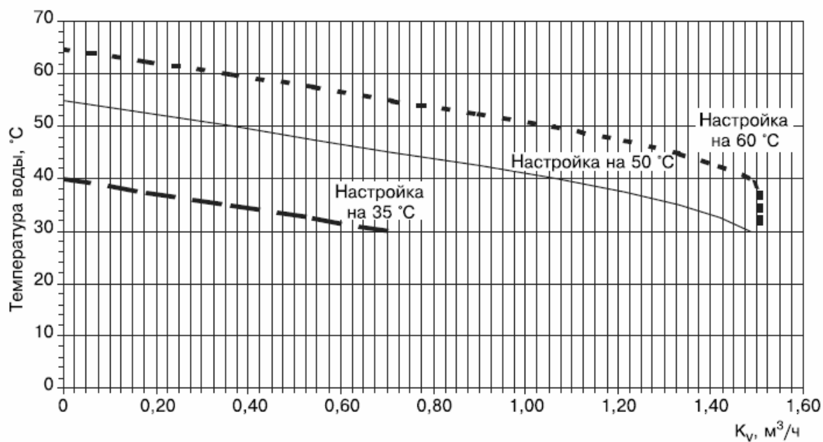
Рис. 6. Зависимость K_v клапана МТСV, D_y=15\text{мм} , от его настройки и температуры воды. (Взято из RC.08.A6.50)
